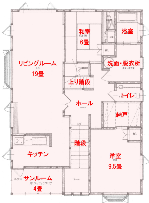
2階 114.27㎡
