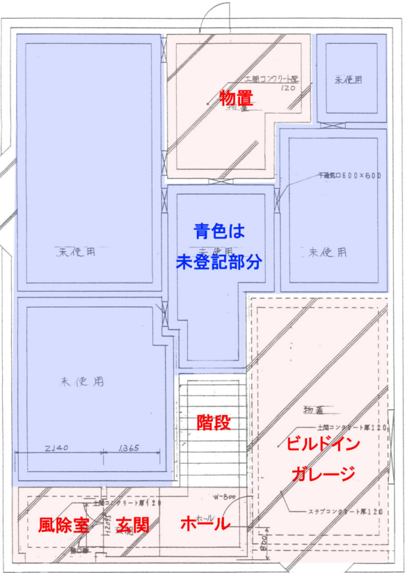
1階 45.13㎡
