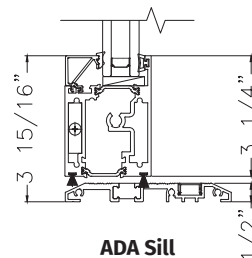
ADA Sill
