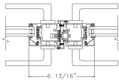
Astragal
