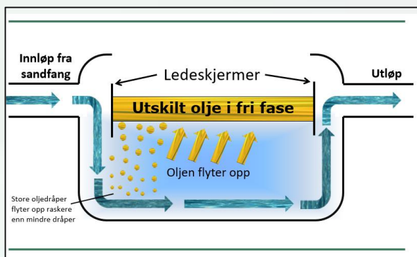
Figur 1: skematisk beskrivelse av hvordan en oljeutskiller virker
