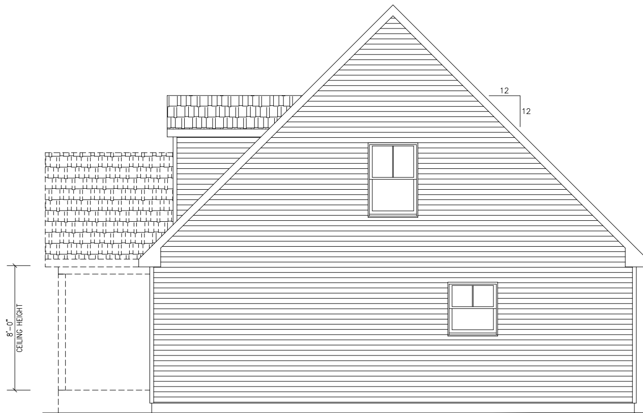
RIGHT ELEVATION
