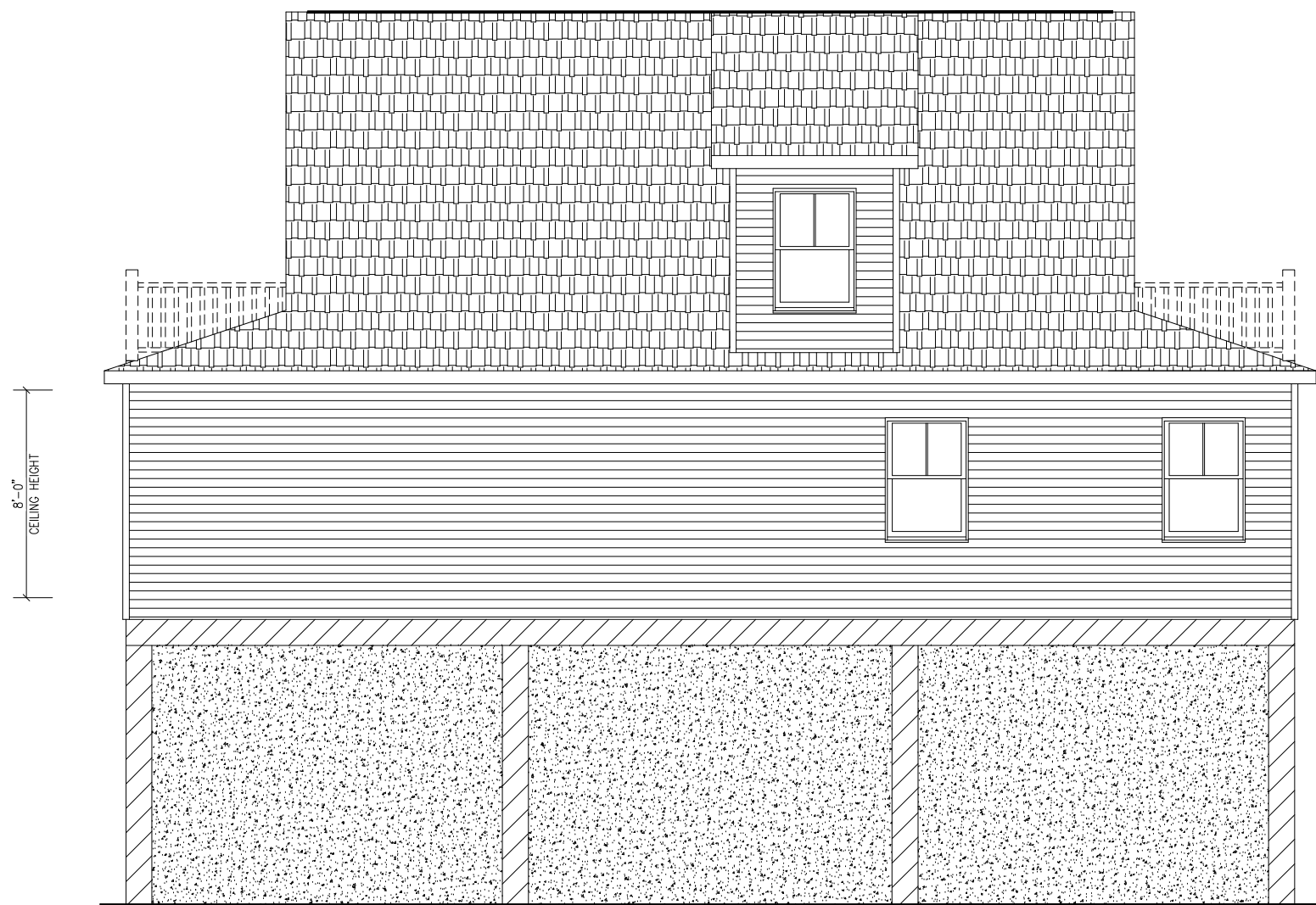
RIGHT ELEVATION
