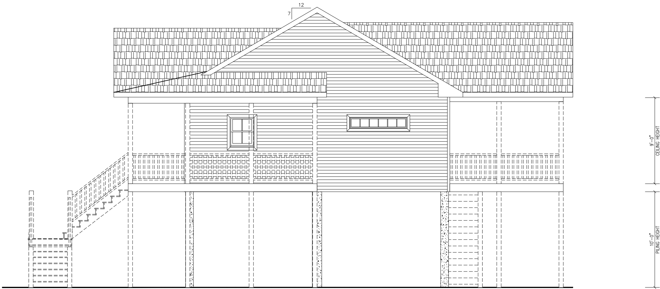
RIGHT ELEVATION
