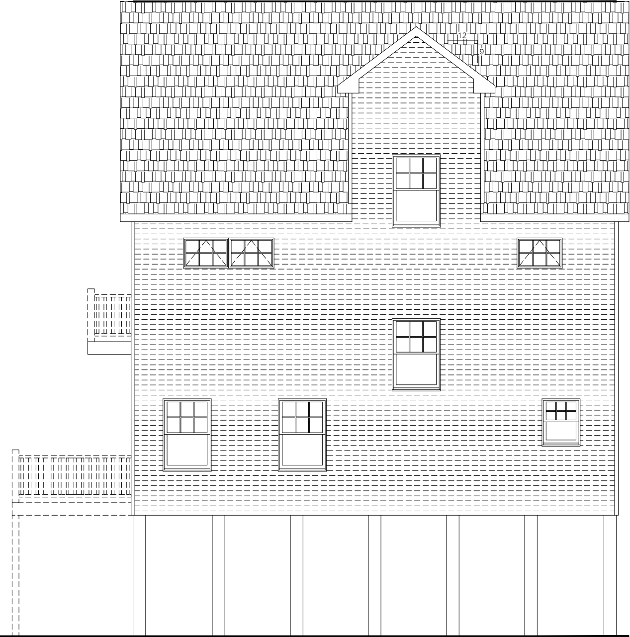
RIGHT ELEVATION
