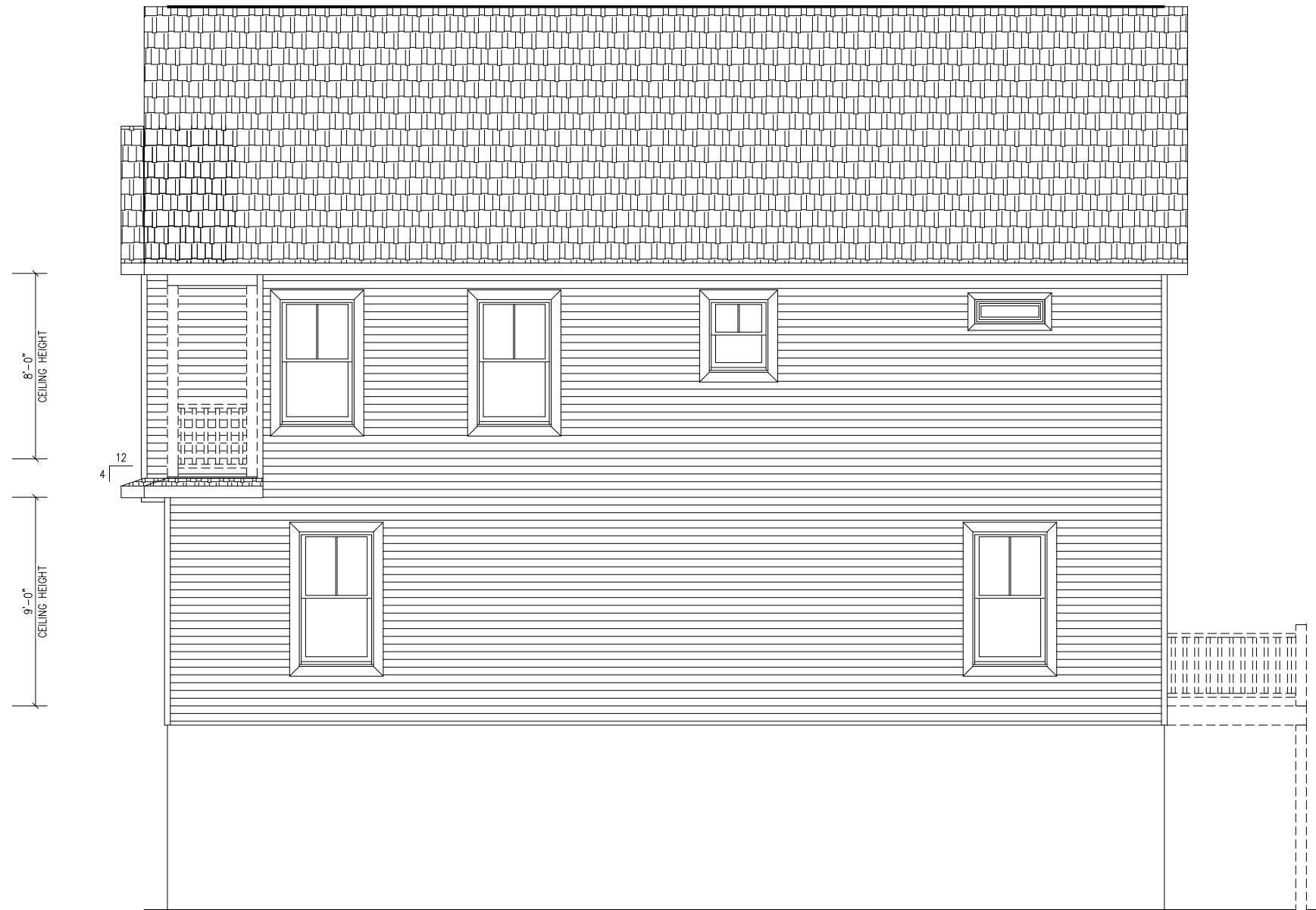
RIGHT ELEVATION
