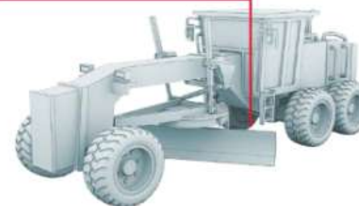
Konfiguration eines Dual-Laserempfängers
