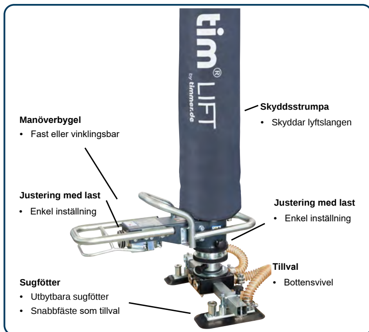
Variabelt manöverhandtag
