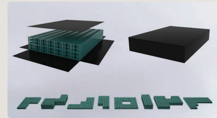
Modulare Regenwasser-Speicher-Rigolen.
