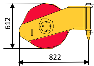
臂端单滑轮 107kg Single top
