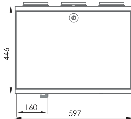
L-malli edestä
