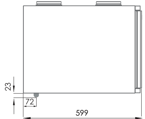
L/R-malli sivusta
