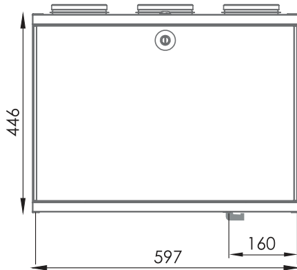
R-malli edestä
