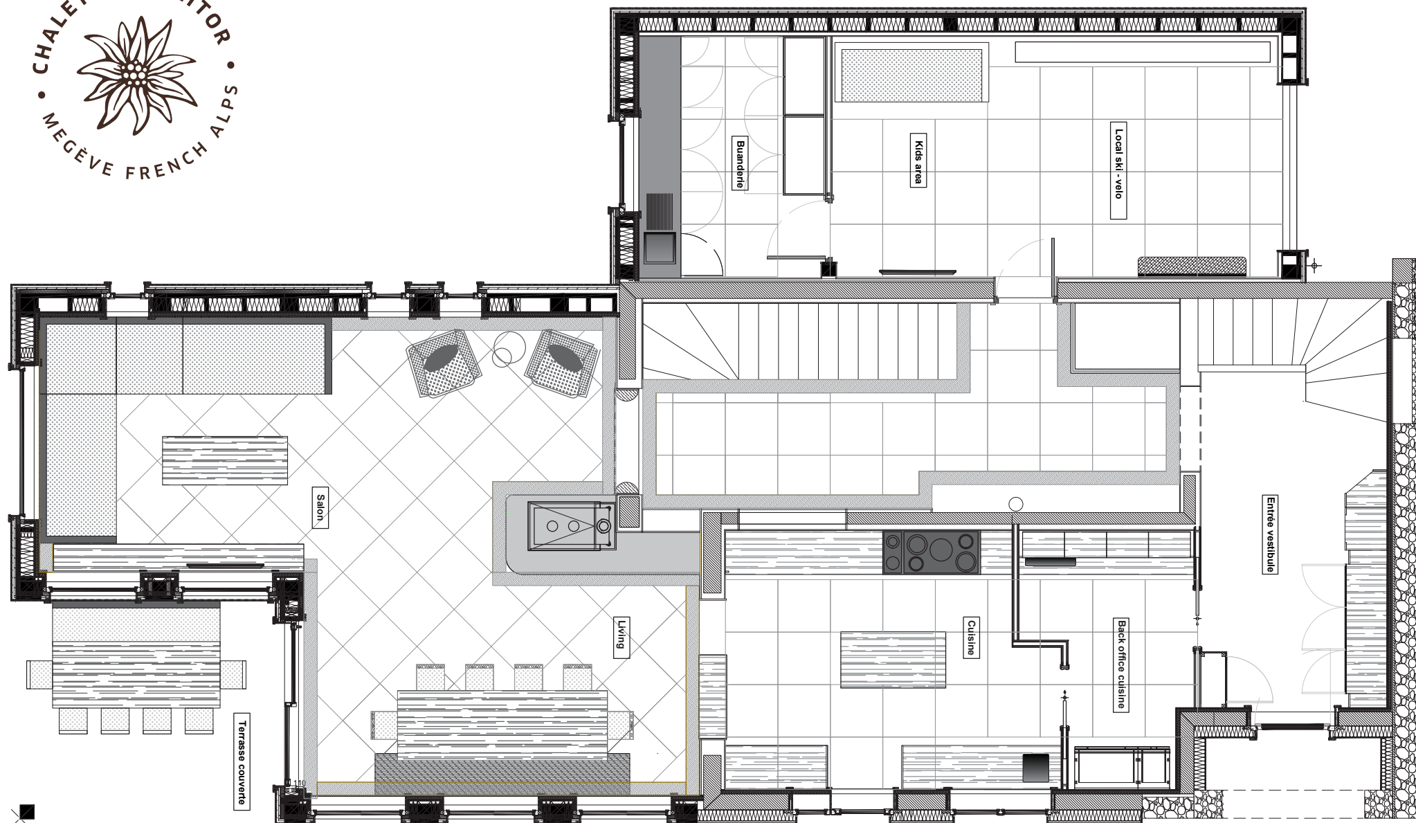
CHALET LE MOLITOR . REZ DE CHAUSSÉE
