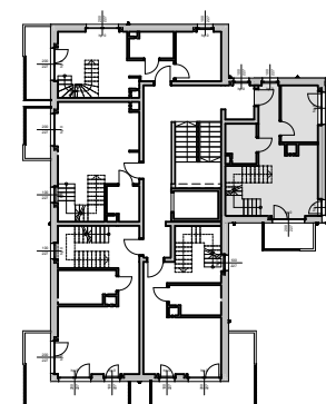
SCHEMAT KONDYGNACJI
