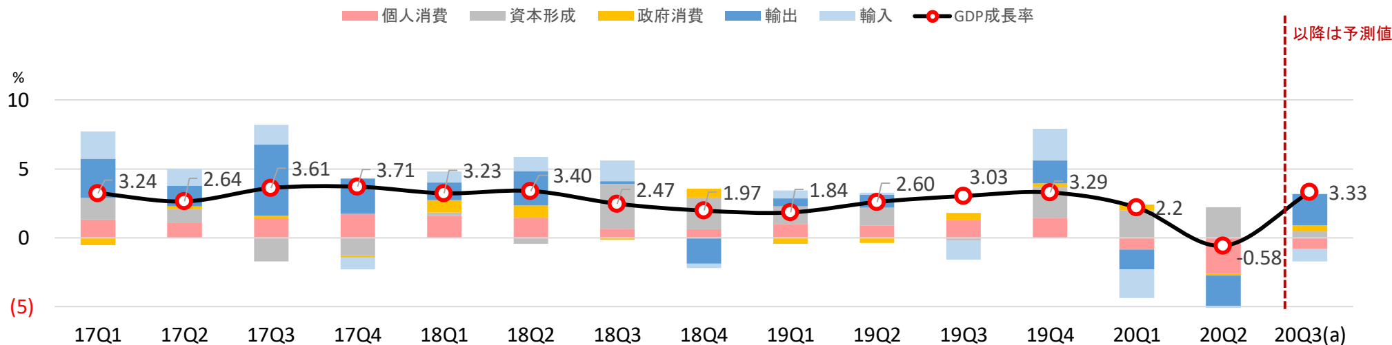
台湾の実質GDP成長率(前年同期比)と各項目の寄与度
