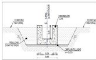
Figura 91. Perfil tipo de bocaneta (Fuente: Arcadis, 2021)
