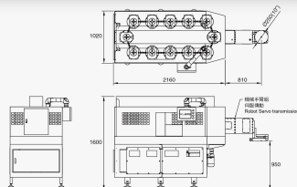
側進式交換工作站 Lateral feeding workstation
