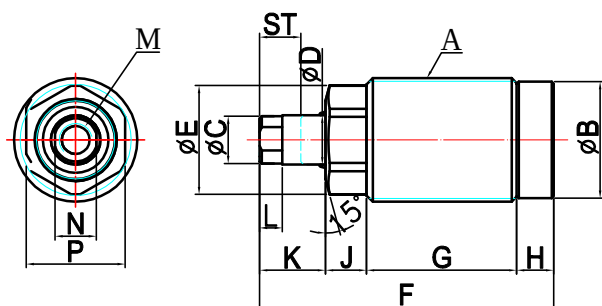
外型尺寸
