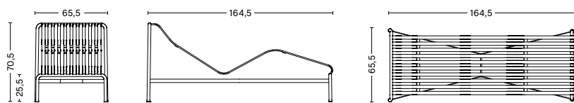
PALISSADE CHAISE LONGUE Width 65,5 cm Depth 164,5 cm Height 70,5 cm Seat height 25,5 cm Weight 22,5 kg
