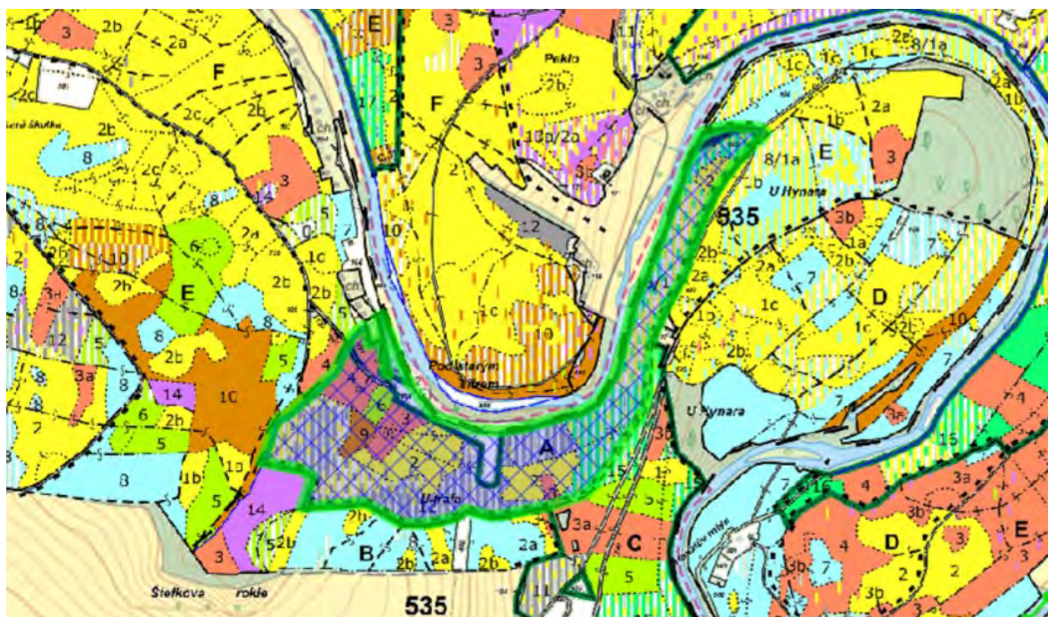
Obrázek č. 3: Výřez porostní mapy s vyznačením lokality – ostrova obnovy „U Hynara“
