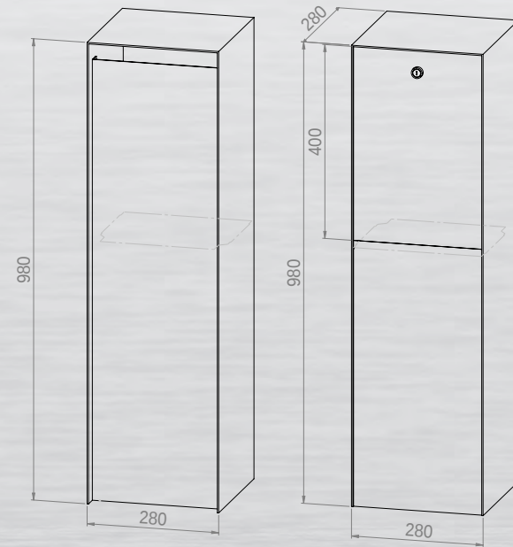
Colum met pakjesbus
