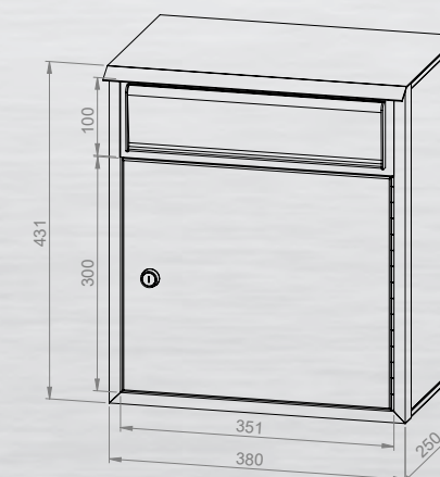
T11 Inwerpopening: B 300 x H 50 mm
