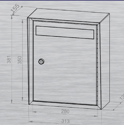
R11 Vlak Inwerpopening: B 250 x H 40 mm
