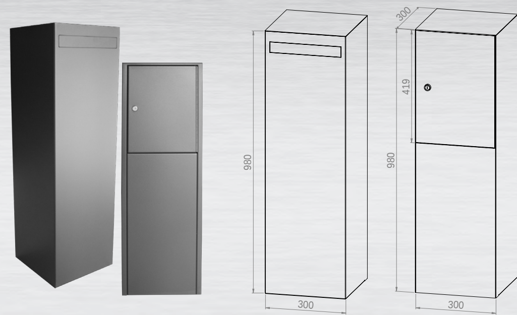
Pilast met pakjesbus
