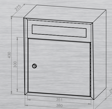
T11 Egale Ouverture: L 300 x H 50 mm
