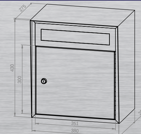
T11 Vlak Inwerpopening: B 300 x H 50 mm
