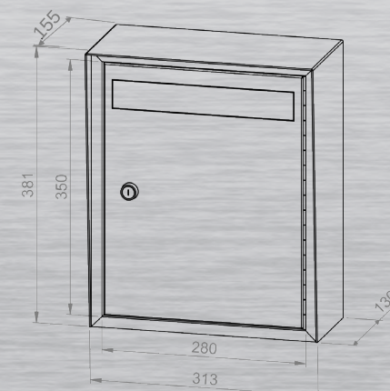
R11 Egale Ouverture: L 250 x H 40 mm
