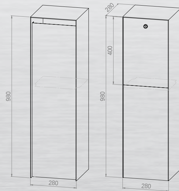
Colum avec boîte pour colis
