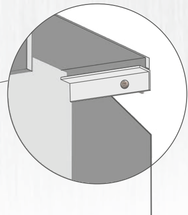
BEVESTIGING IN PARLOFOONVAK
