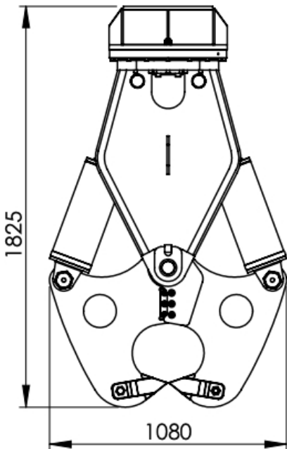
vooraanzicht/front view/ Vorderansicht/vue de face
