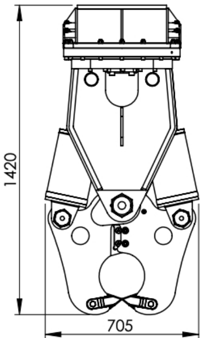
vooraanzicht/front view/ Vorderansicht/vue de face
