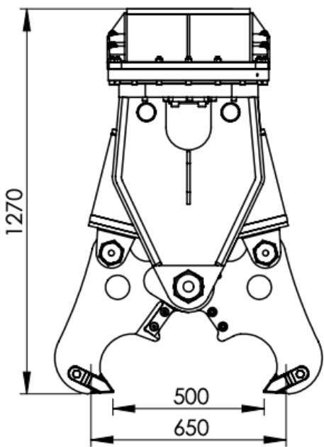
zijkant/side view/ Seitenansicht/vue de côté
