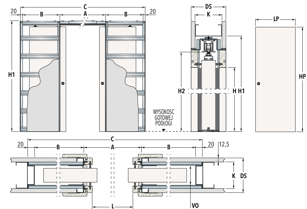
WYMIARY KASETY STANDARDOWEJ
