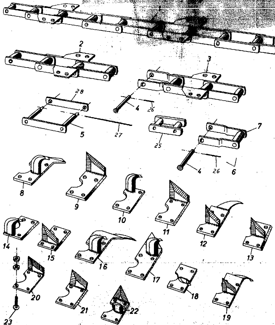
Übersicht der Fräskette mit Werkzeugen
