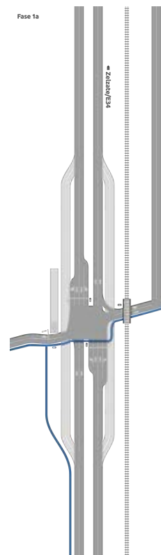
Bouw dakplaat fietsonderdoorgang, toegangshelling en voorbereiding op-en afritten. Lokaal verkeer via tijdelijke weg rond bouwuip.
