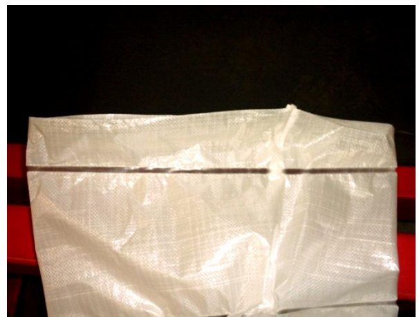
Märkning av storsäck med printern, t ex batchnr, vikt mm.
