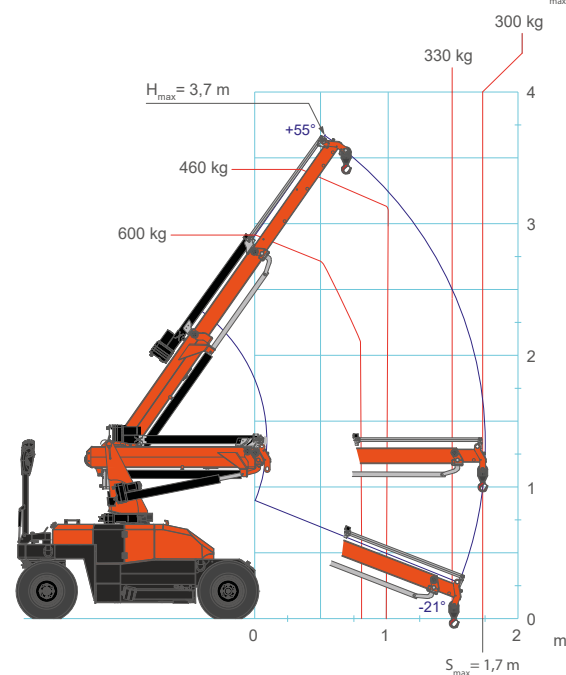
Haken-Lastdiagramm
