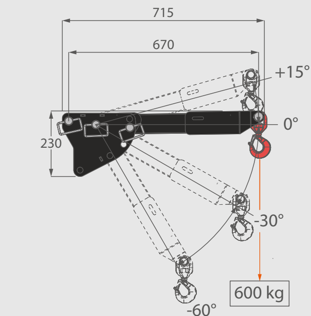
Säulenschwenkhaken- Lastdiagramm
