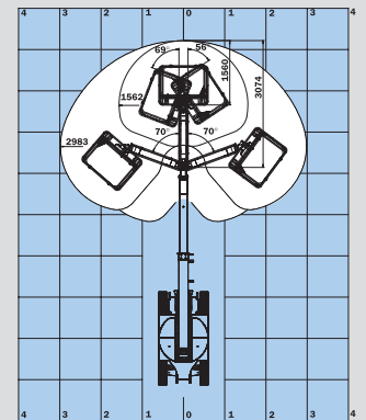
Option 3D: Drehung des Schwenkarms
