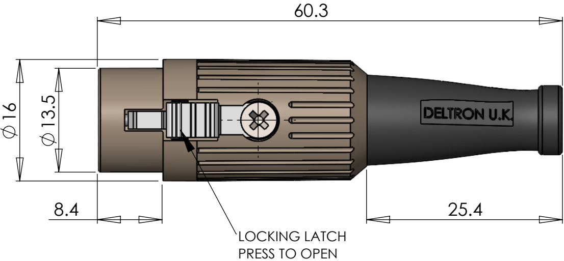
DIMENSIONS
