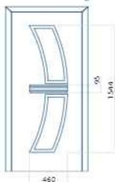
Technische Zeichnung
