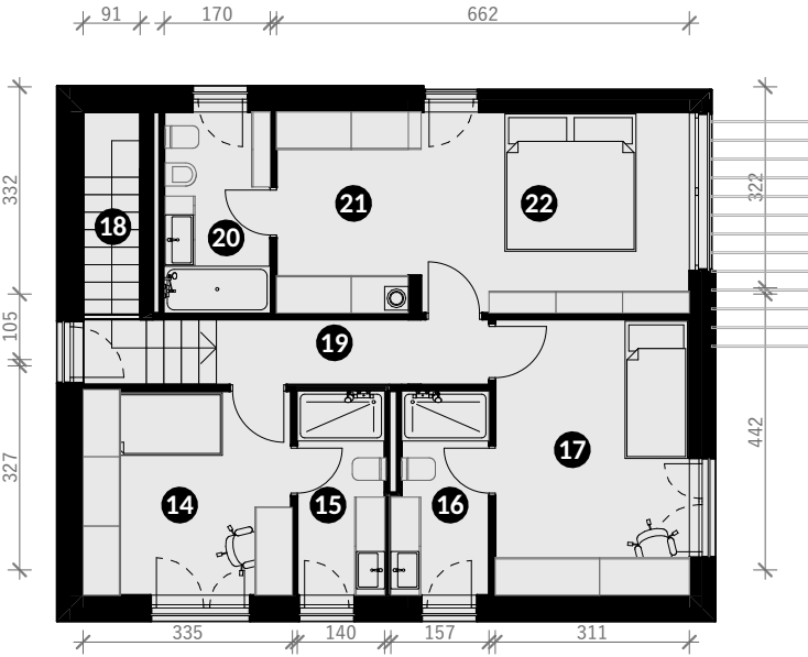
1. KAT
