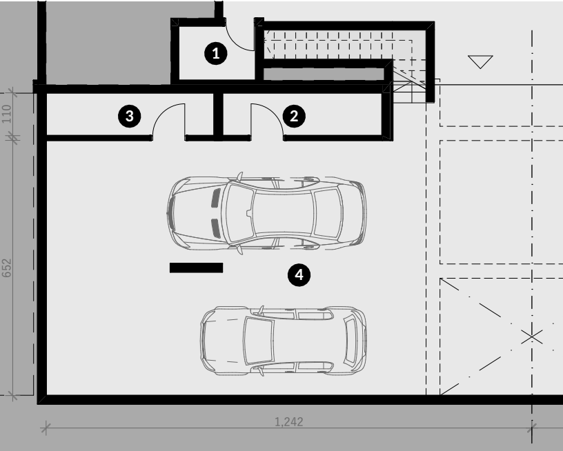
PODRUM
