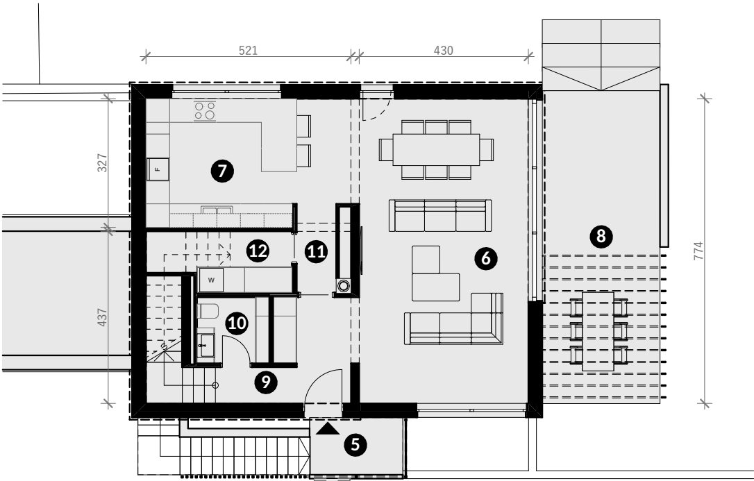
PRIZEMLJE
