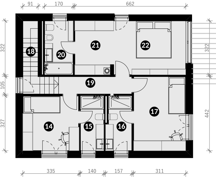
1. KAT
