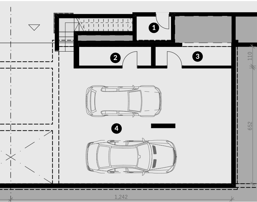
PODRUM
