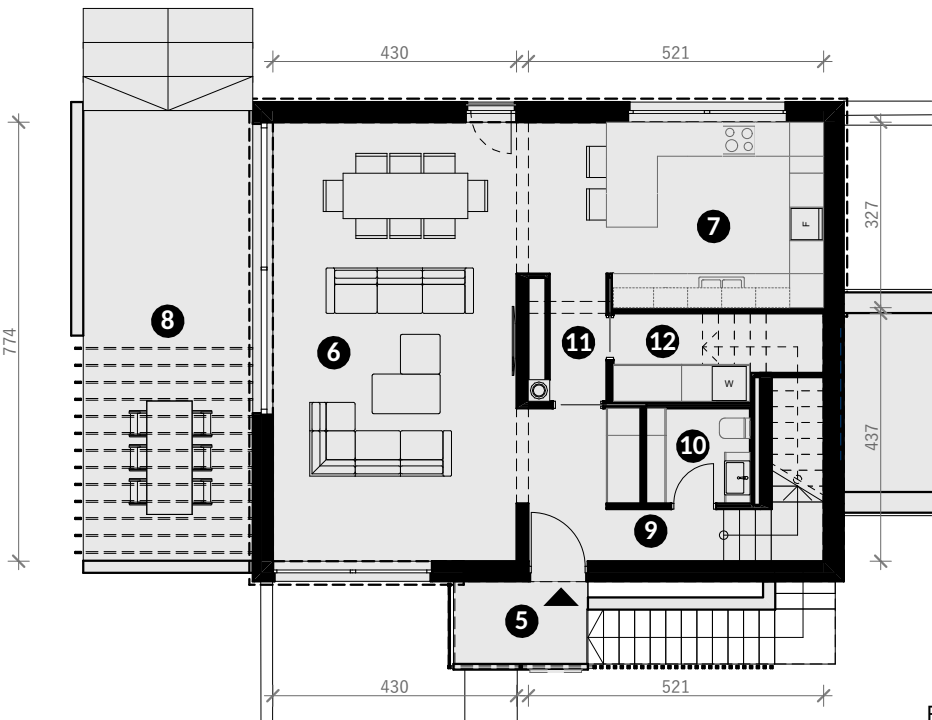
PRIZEMLJE
