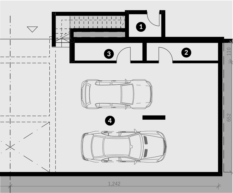
PODRUM
