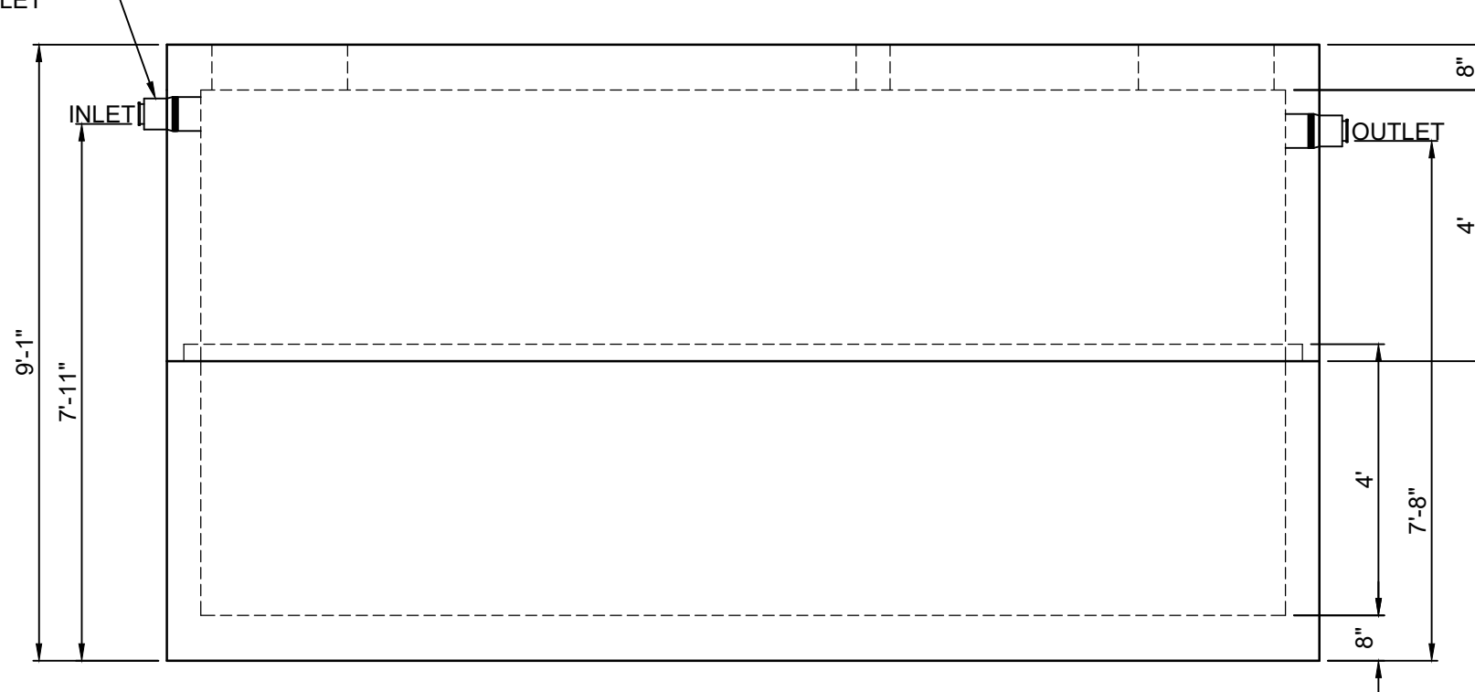
SECTION VIEW SCALE: 3/8" = 1'-0"
