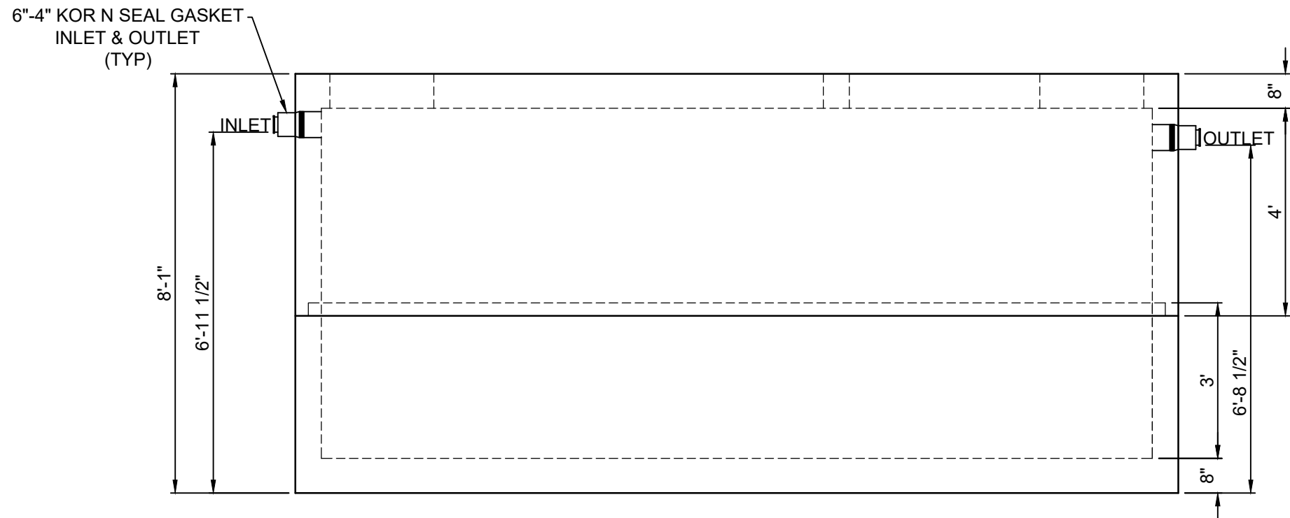
SECTION VIEW SCALE: 3/8" = 1'-0"
