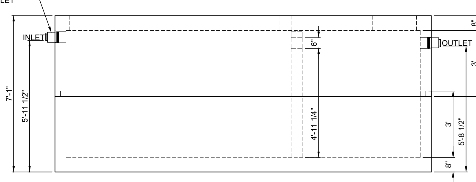
SECTION VIEW SCALE: 3/8" = 1'-0"
