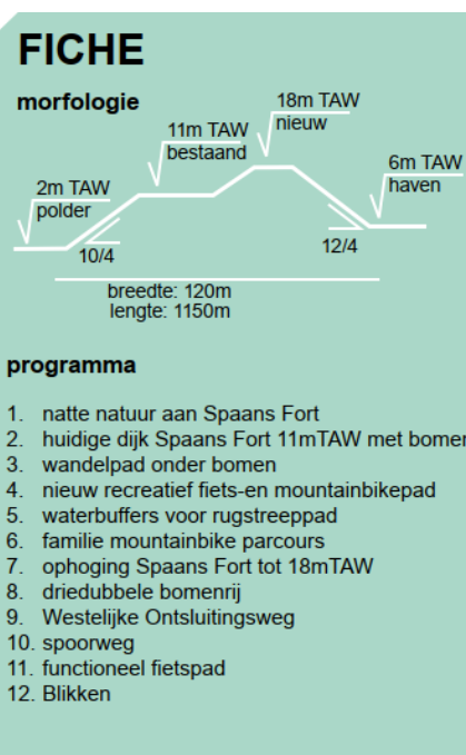
Figuren. Ontwerp 2D Spaans fort en schematische fiche (Bron: Masterplan Bufferlandschap ECA, Omgeving, januari 2023)
