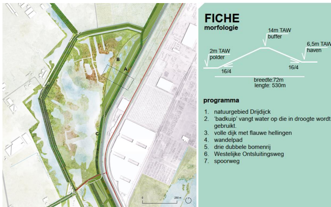
Figuren. Ontwerp 2D Drijdijk en schematische fiche (Bron: Masterplan Bufferlandschap ECA, Omgeving, januari 2023)
