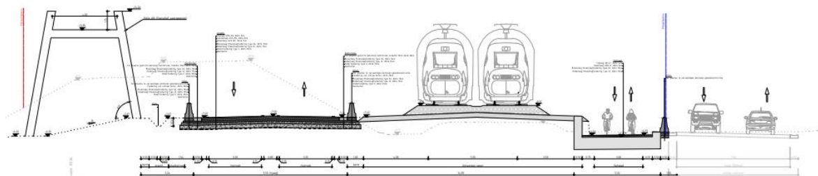
Figuur. Dwarsprofiel (H) Westelijke Ontsluiting net ten zuiden van Putten Hoog richting TGD (Bron: SBE)
