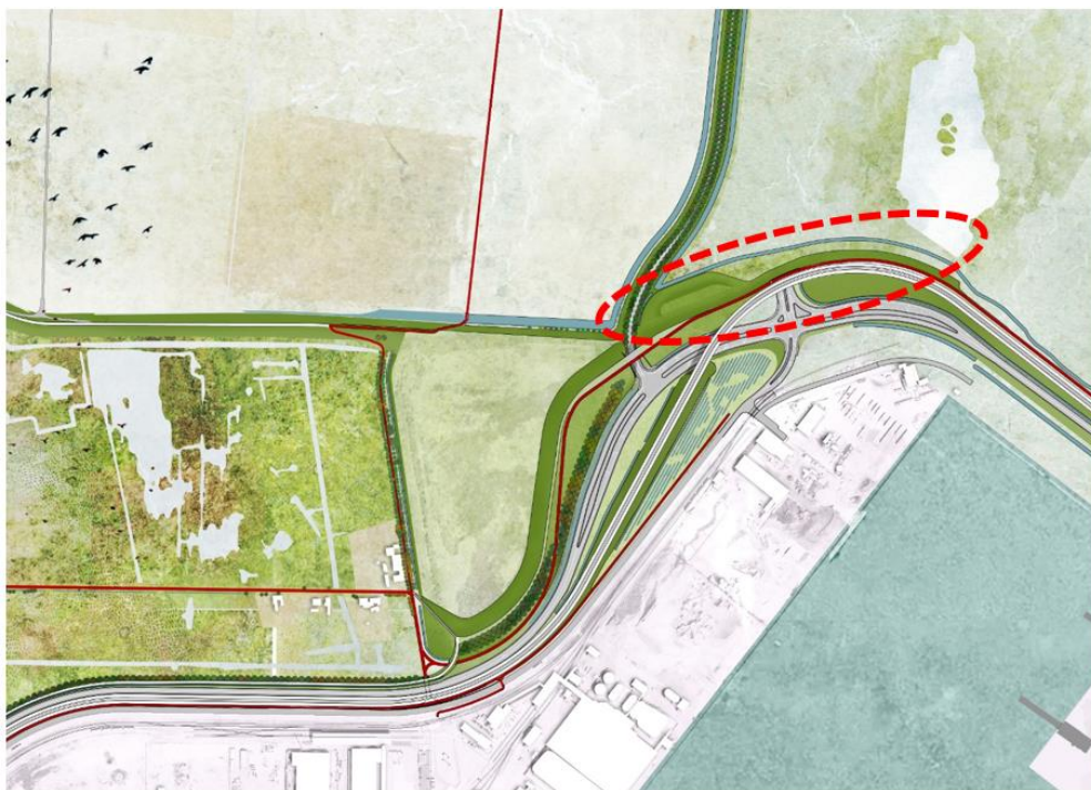
Figuur. Polderheuvel tijdens stap 1, met aanduiding van de situering van de tijdelijke buffer (Bron: Omgeving, april 2023)
