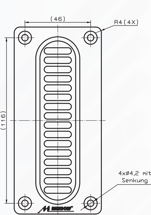
Ansicht Vorne
