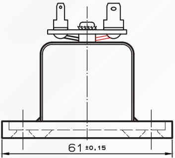
Draufsicht
