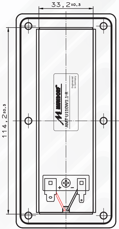
Ansicht Hinten
