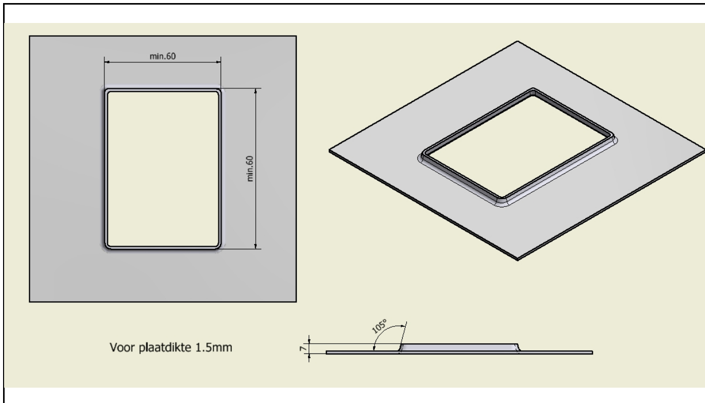
Flanging tool upwards rechte zijde
