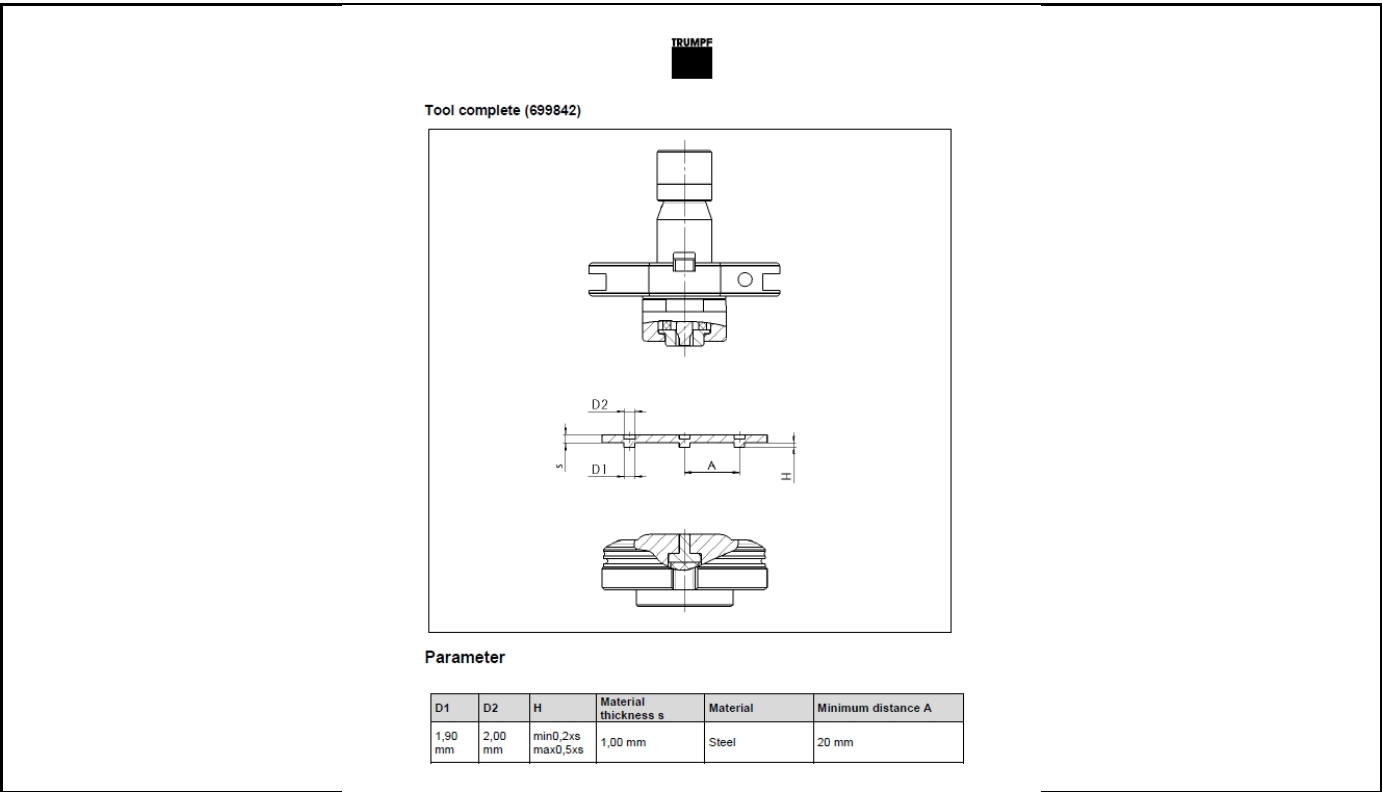
Centreerpunt 2 down
