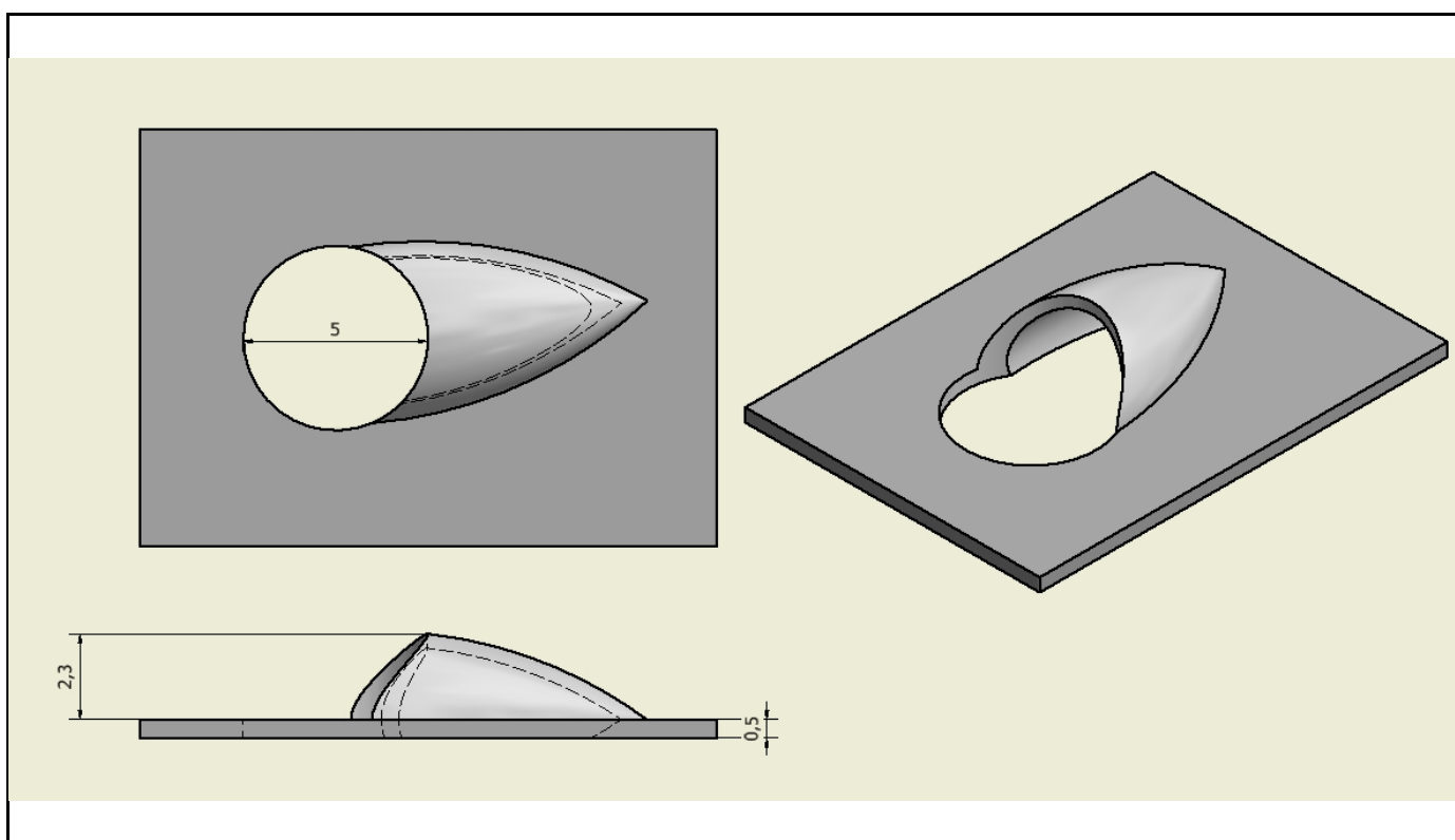
Embossing tool upwards voor 0.5mm
