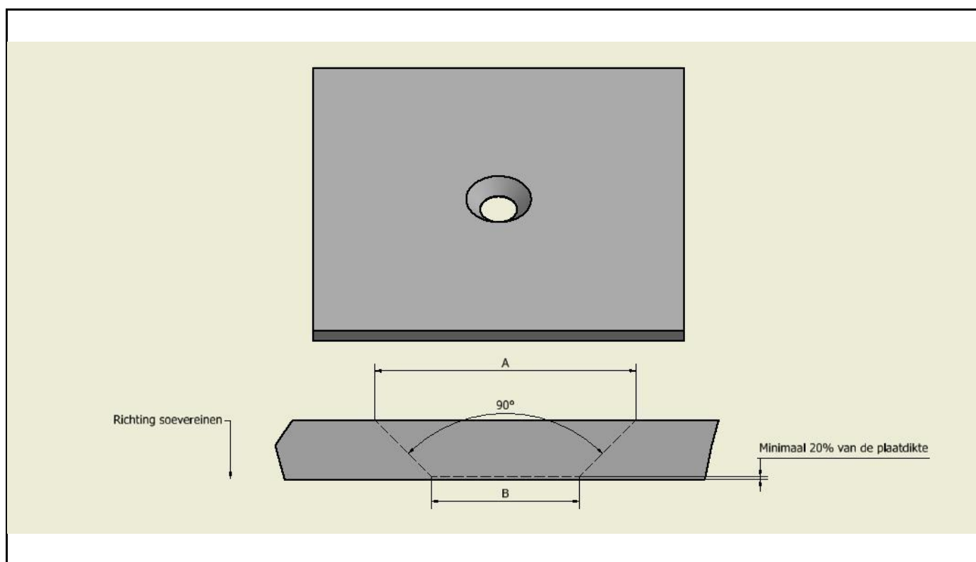
Soeverein downwards Ø6.2 naar Ø3.4 voor 1.5mm
