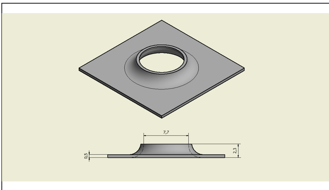
Form upwards extrusion voor 0.5mm
