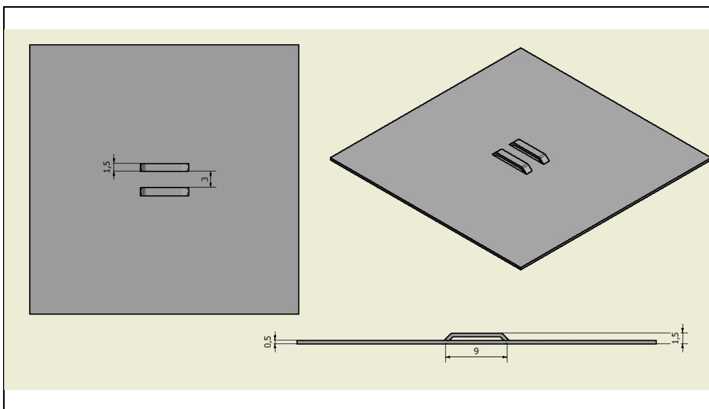
Bridge dubble form downwards voor 0.5mm
