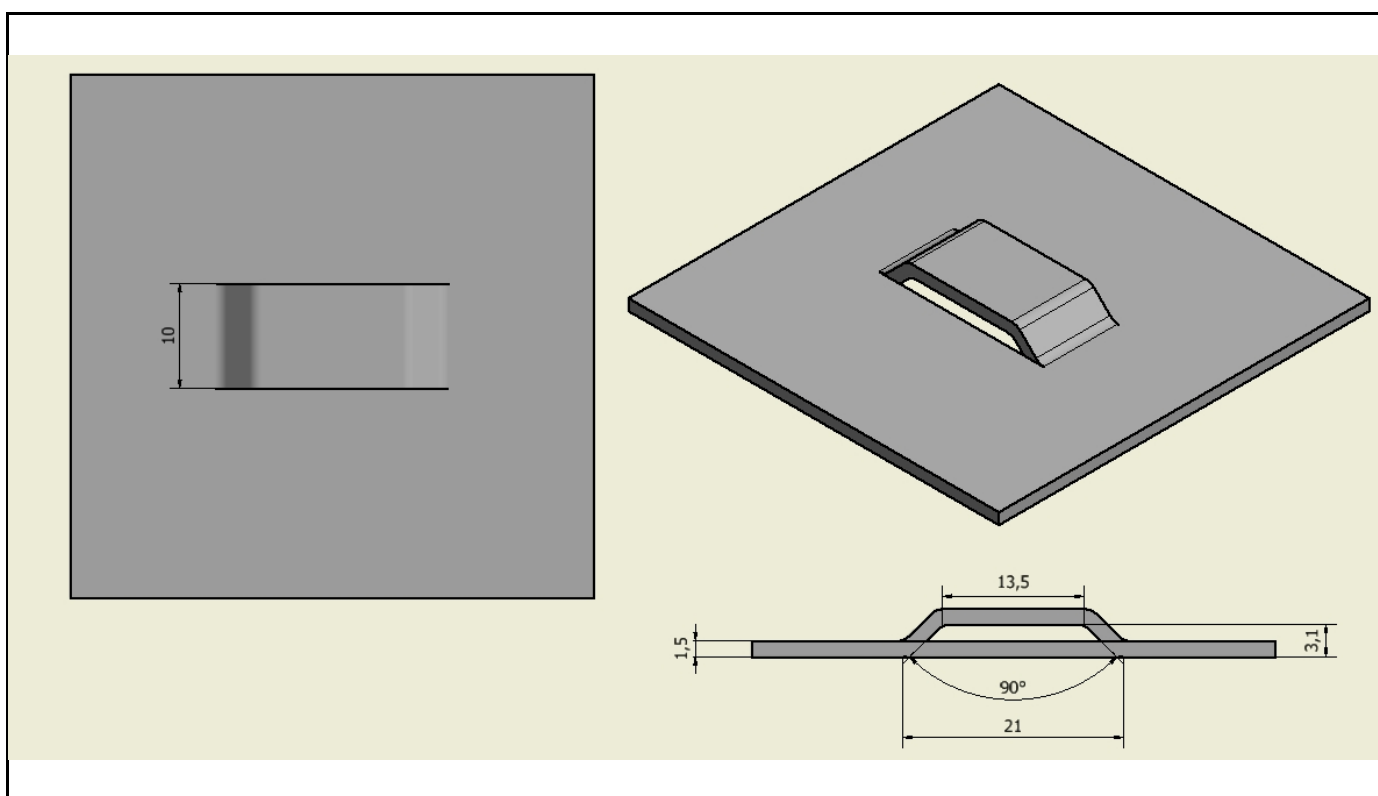
Bridge single form upwards voor 1.5mm
