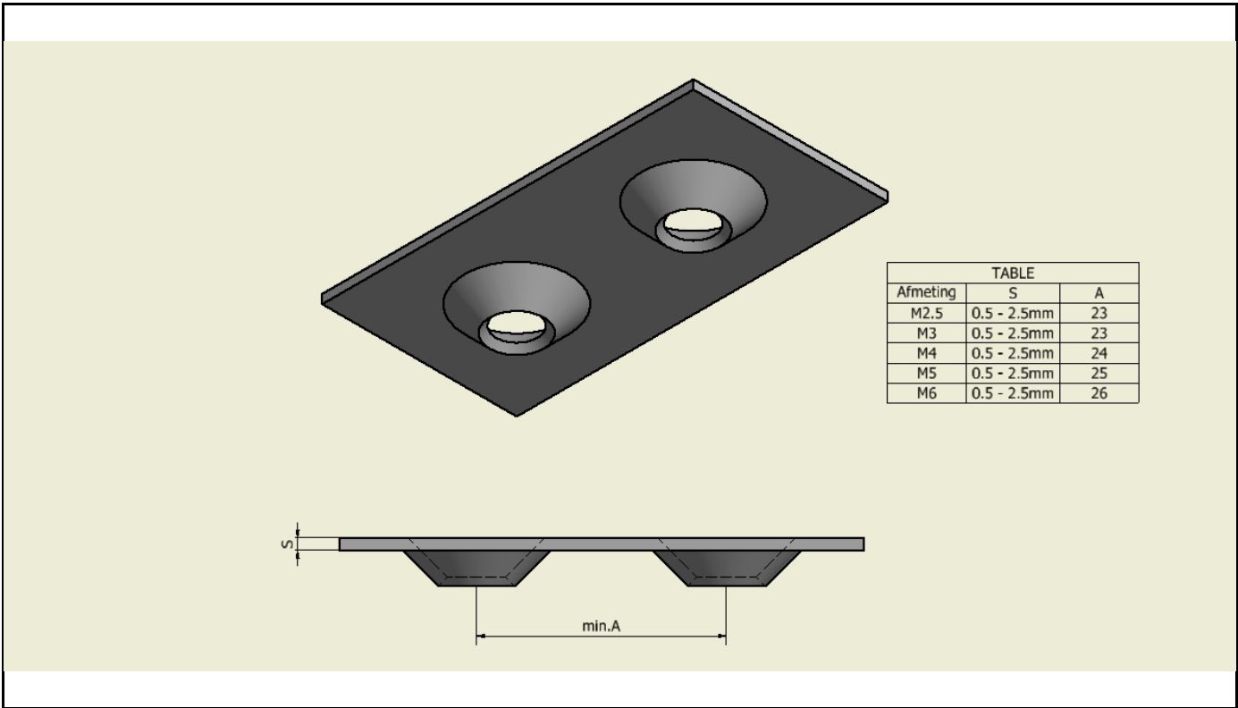
Verzonken doordrukking M4 downwards voor 1.5mm
