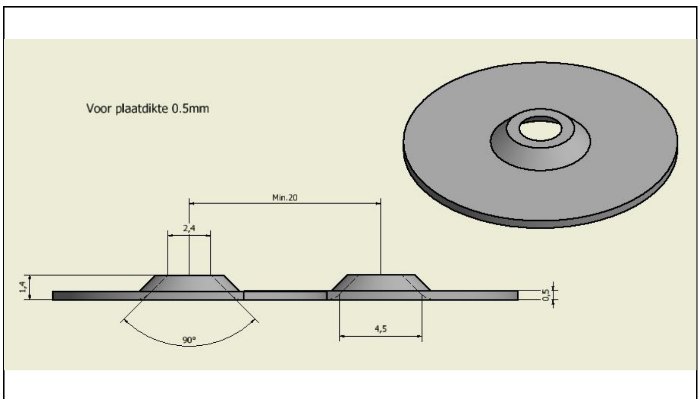
Form countersink tool upwards 4.5 x 2.4 voor 0.5mm
