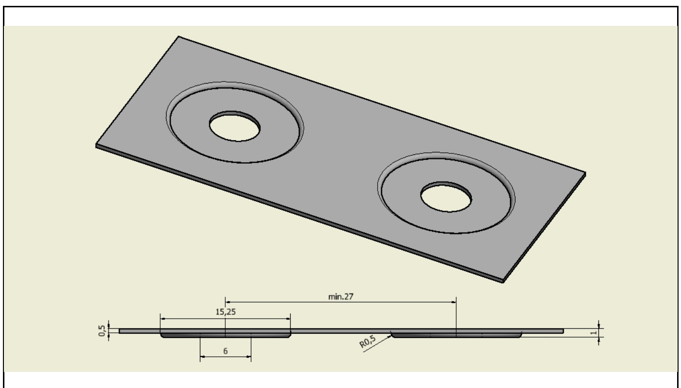
Cup forming tool downwards voor 0.5mm
