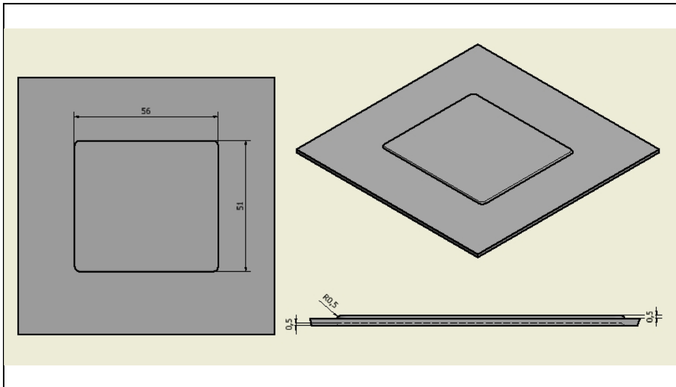
Cup forming upwards 56.0 x 51.0 x 0.5 voor 1.5mm
