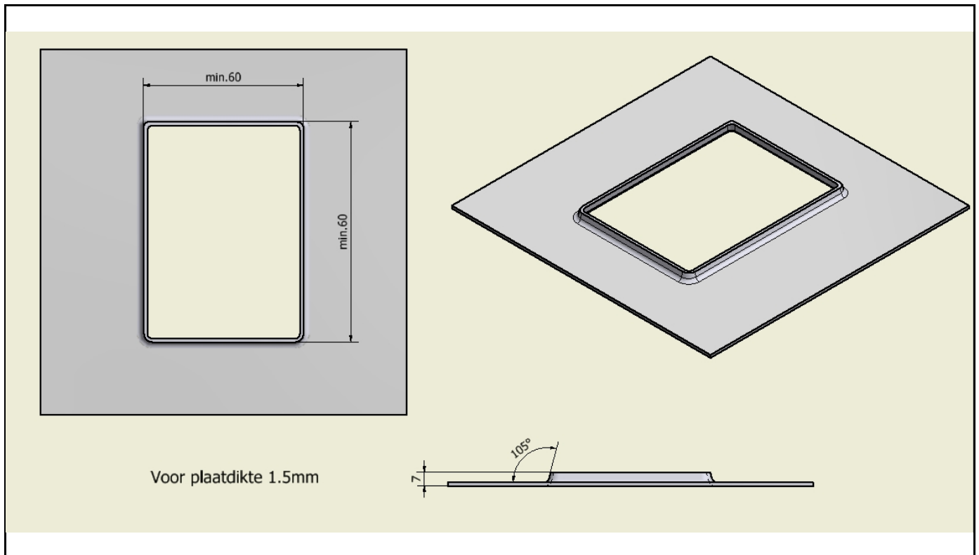
Flanging tool upwards hoeken
