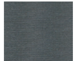
Basalto
