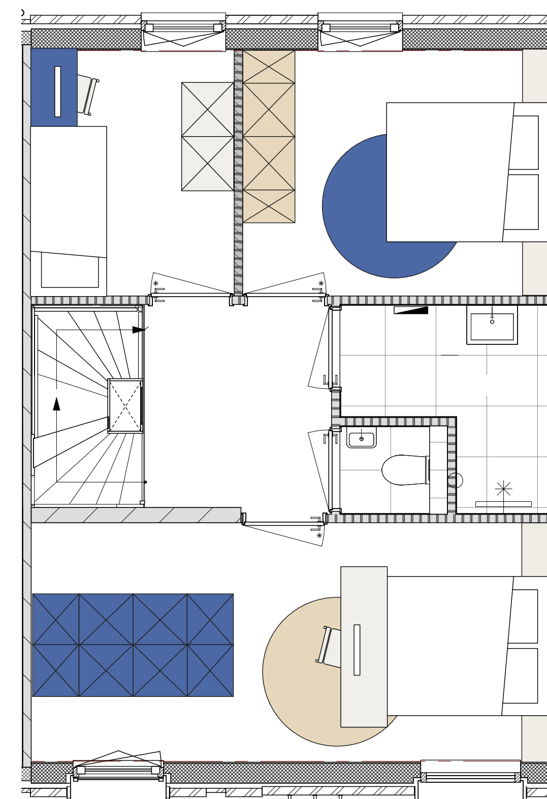
eerste verdieping
