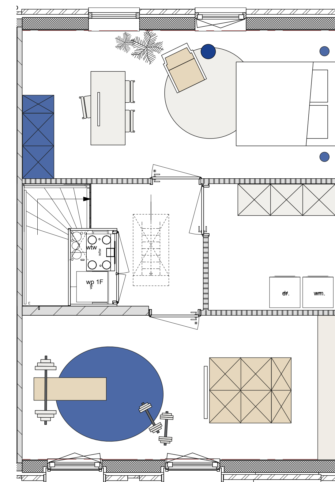
tweede verdieping
