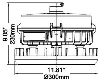
Pendant Mount
