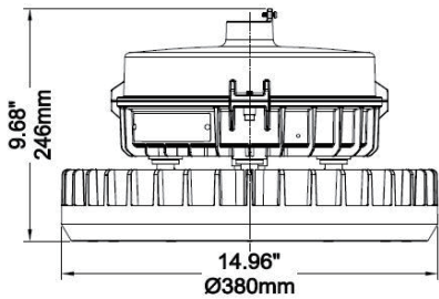
Pendant Mount
