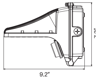
80W(120-347VAC) / 100-120W(120-277VAC&120-347VAC)
