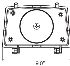
30-60W(120-277VAC&120-347VAC) / 80W(120-277VAC)
