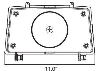
80W(120-347VAC) / 100-120W(120-277VAC&120-347VAC)
