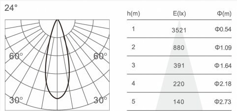
A-Cyl 2 / 24°
