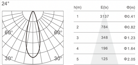
A-Cyl 1 / 24°
