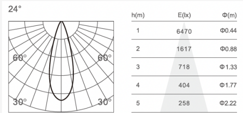
A-Cyl 3 / 24°
