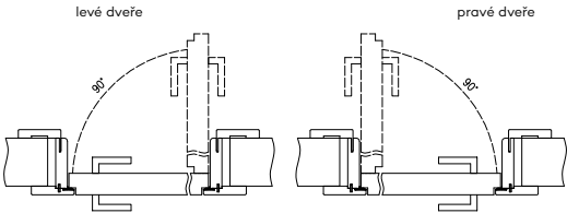
Profil zárubně
