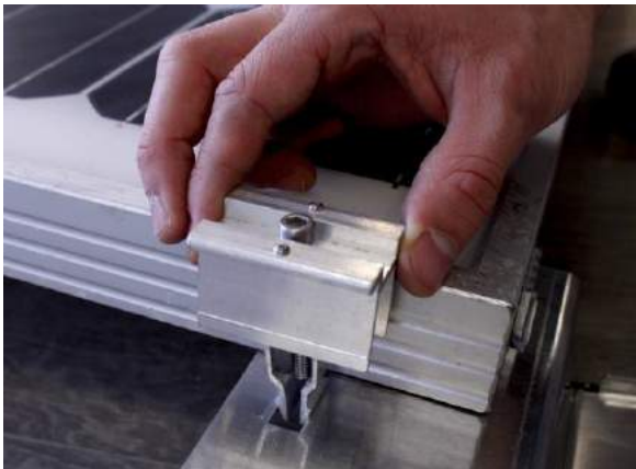
Fig. 10- Click-in KB Konnect Clamp
