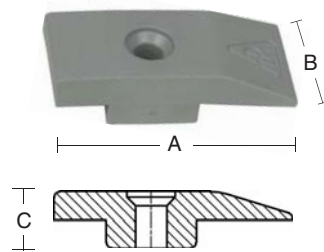
STYREKLODS IPA NR. 63230
