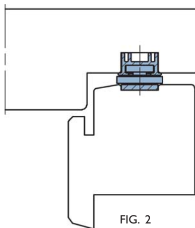
VANDRET SNIT
