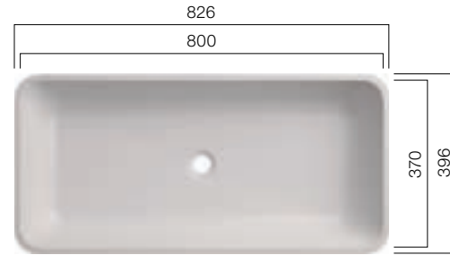
VDS 800.370.R40
