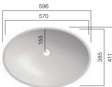
VO 57
