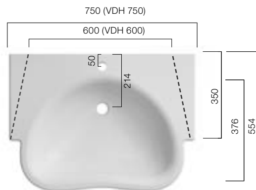
VDH 750 / VDH 600
