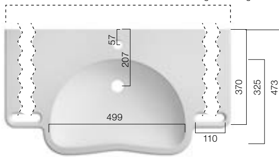
VDH 850 WTH
