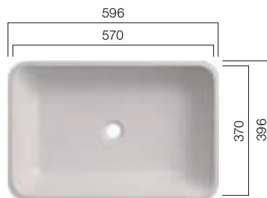
VDS 570.370.R40
