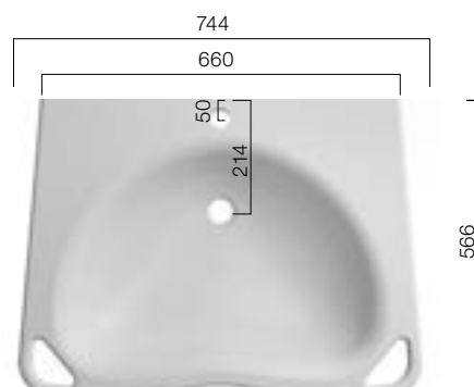
VDH 660
