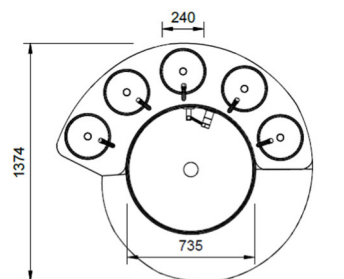
VIVARI@KIDS FOSSI Waschtisch Grundriss
